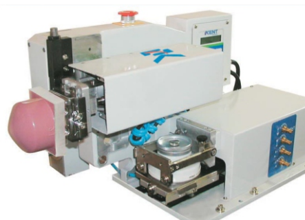
Movimiento giratorio de 90° del tampón
